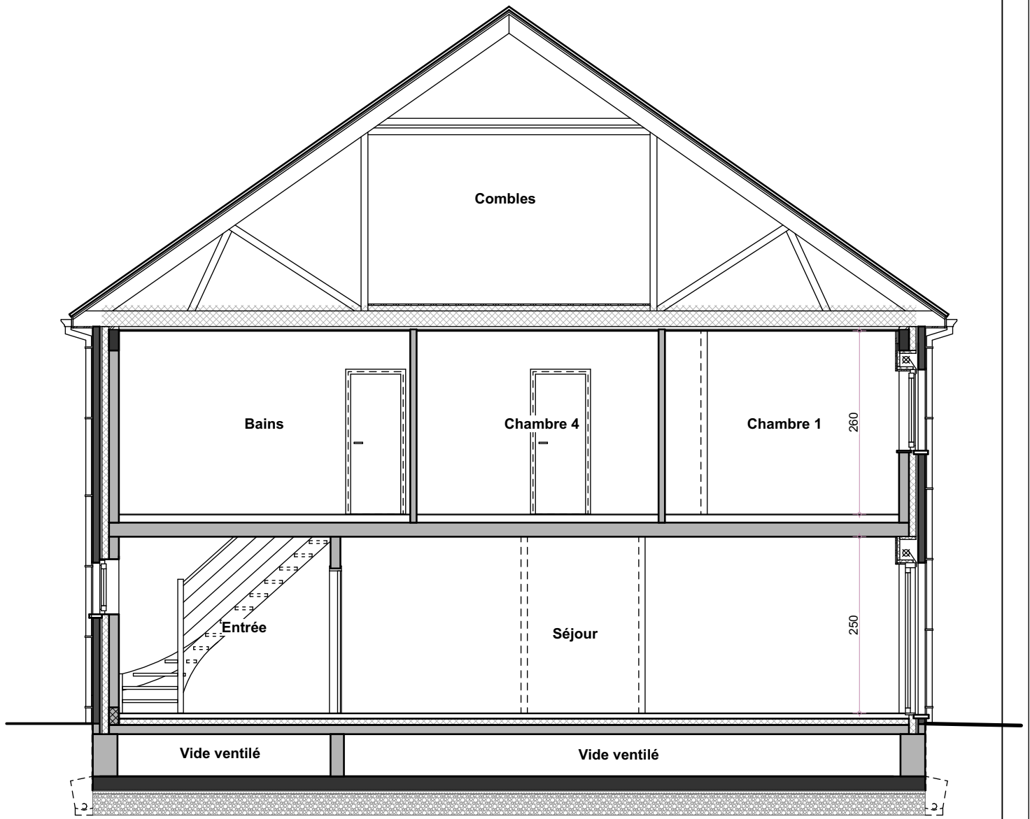
Coupe AA
