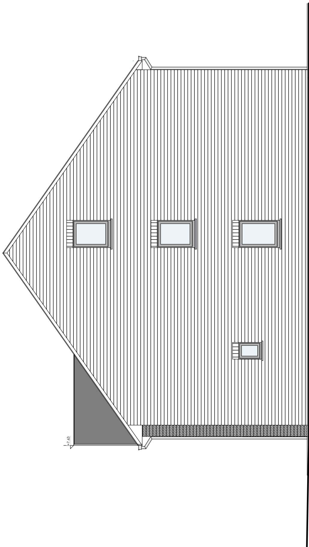
Maison 21 Façade Latérale Droite
