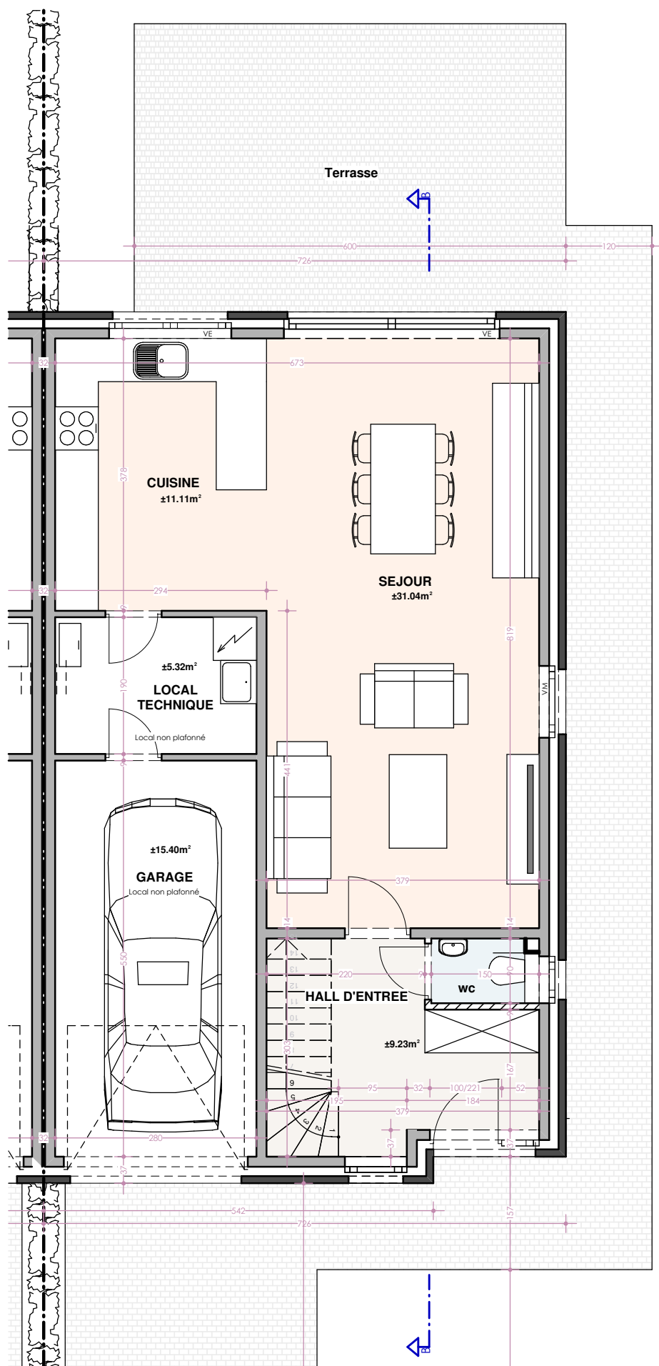
Maison 22 Rez de Chaussée
