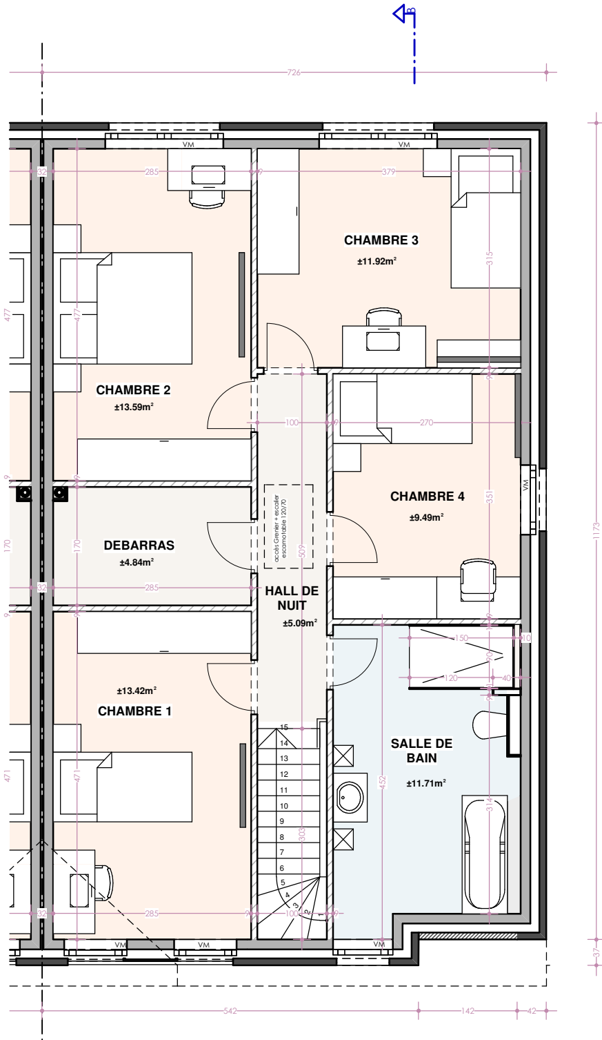
Plan Etage : Maison 22
