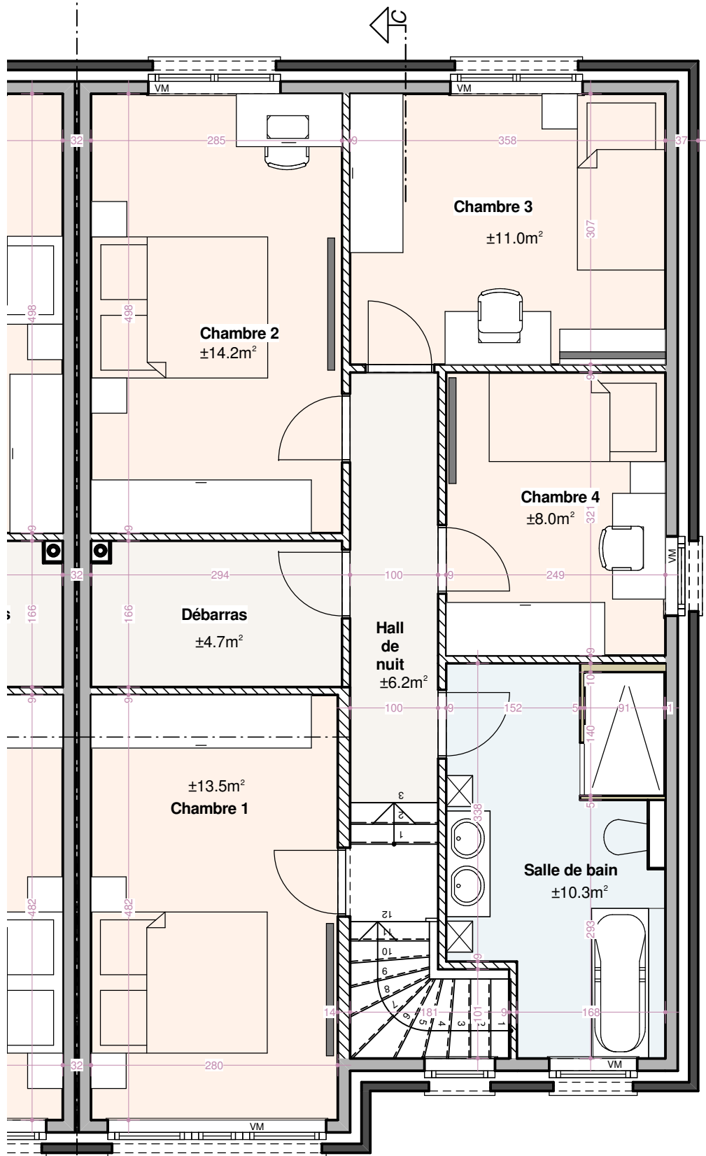
Maison 33/3 : Etage
