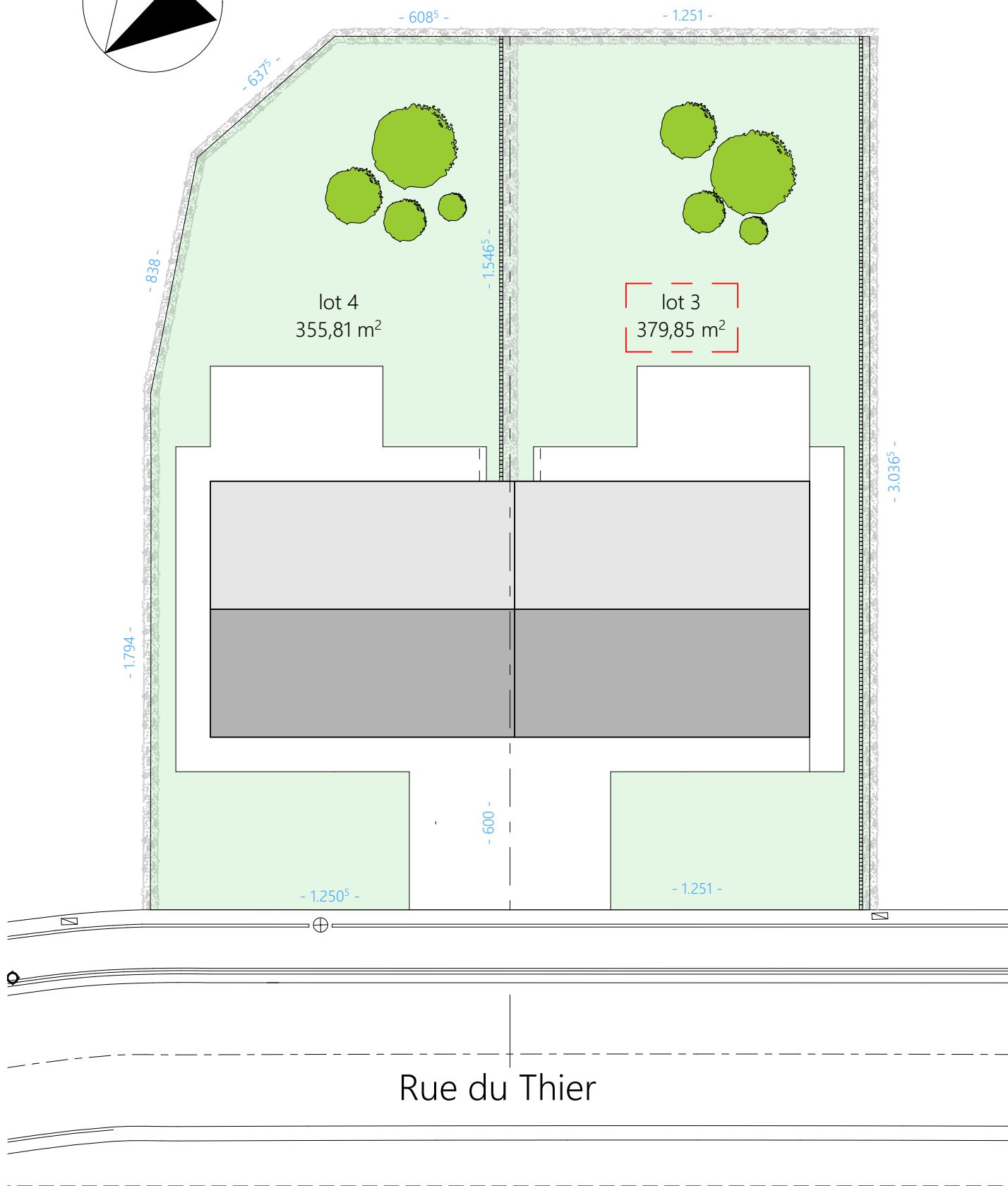
Plan d'implantation
