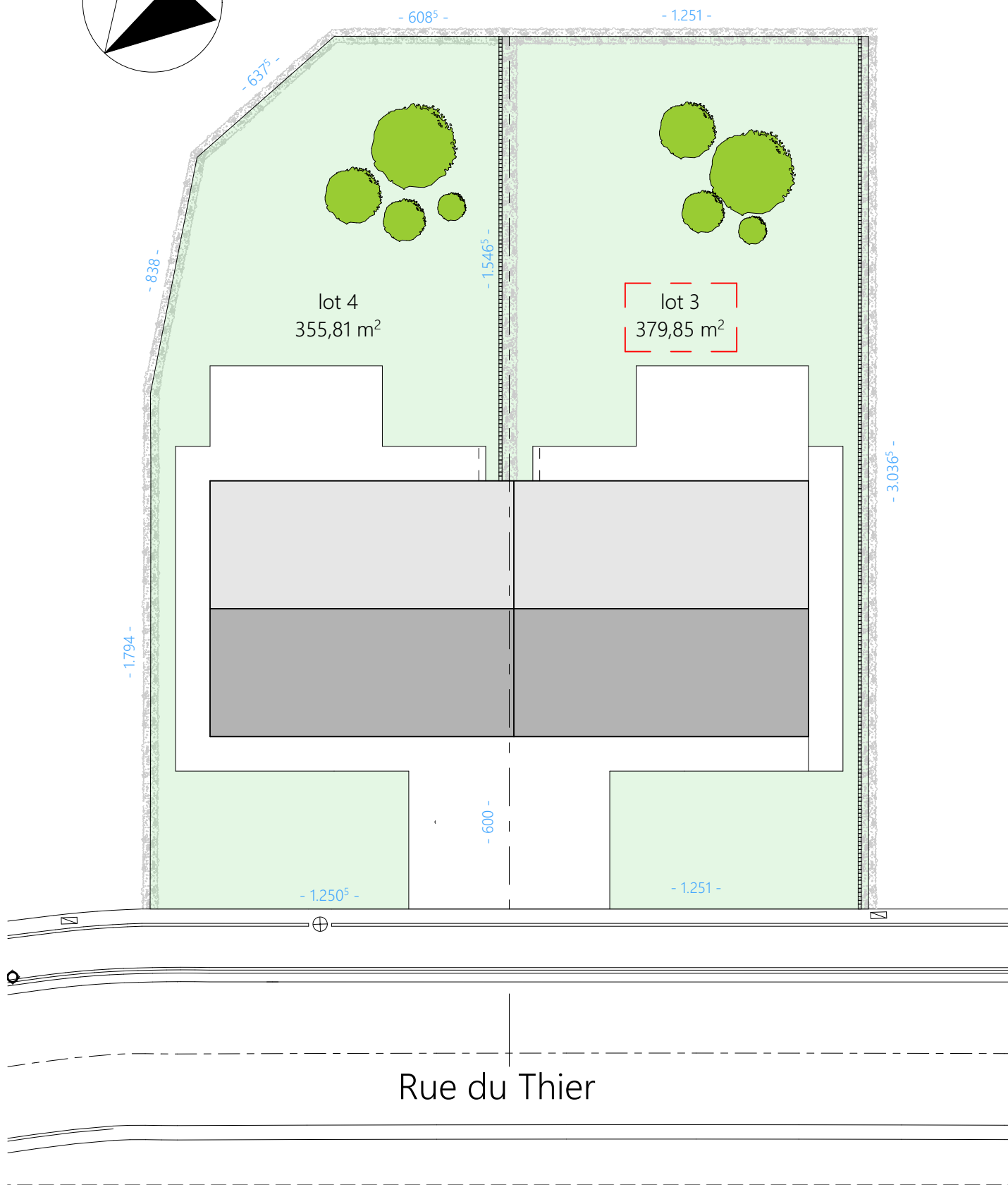
Plan d'implantation
