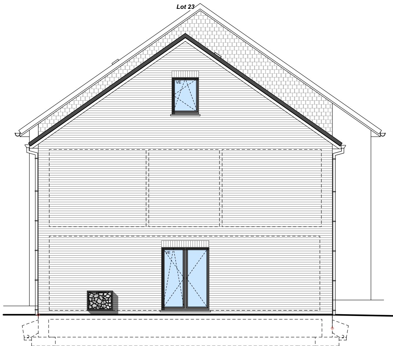
Façade latérale droite
