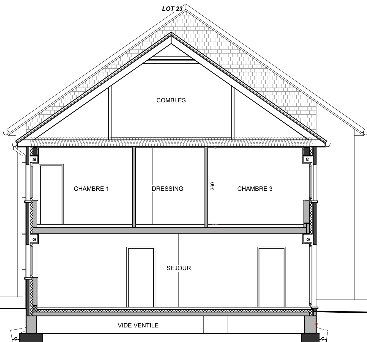
COUPE AA'
