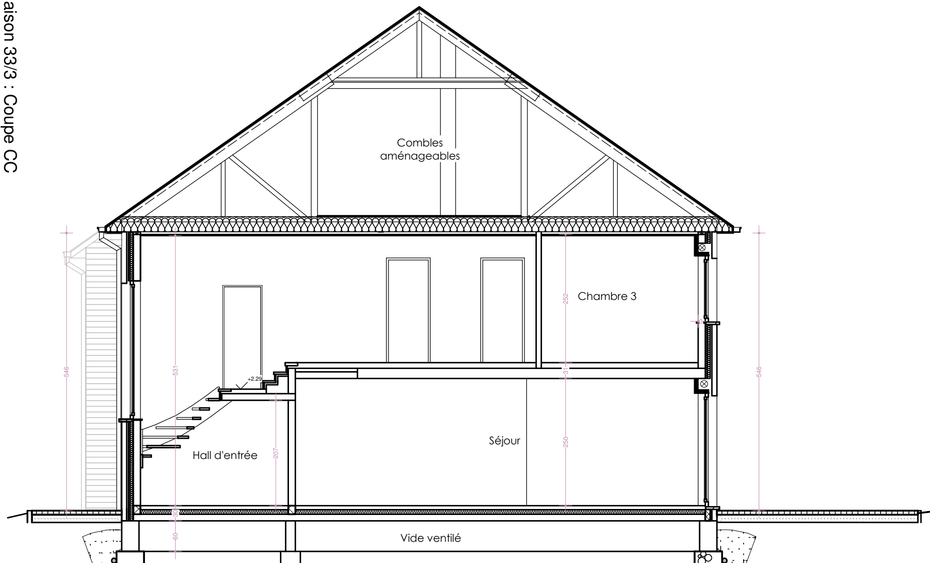
Coupe CC : Maison 33/3
