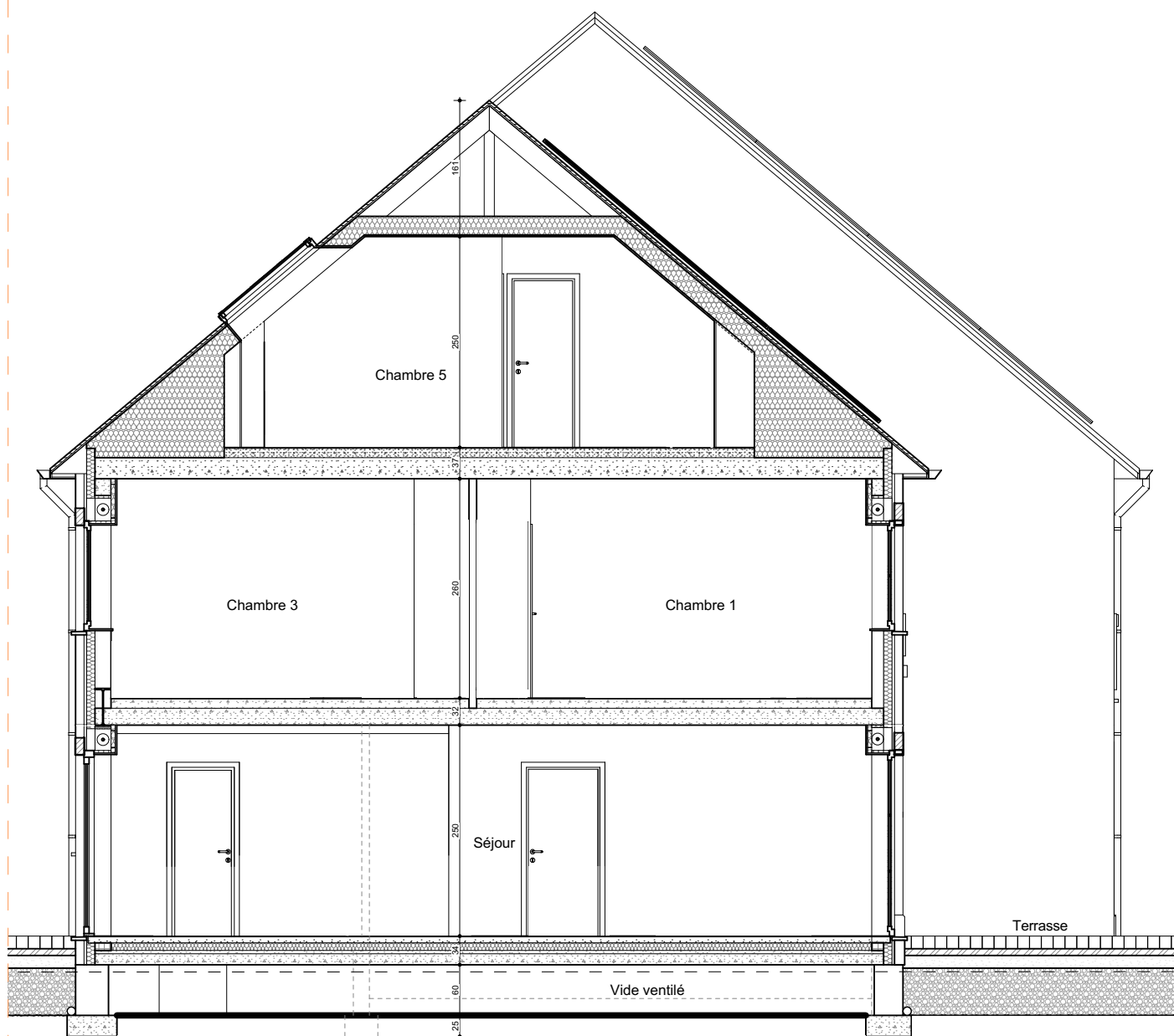
Coupe DD Lot 3
