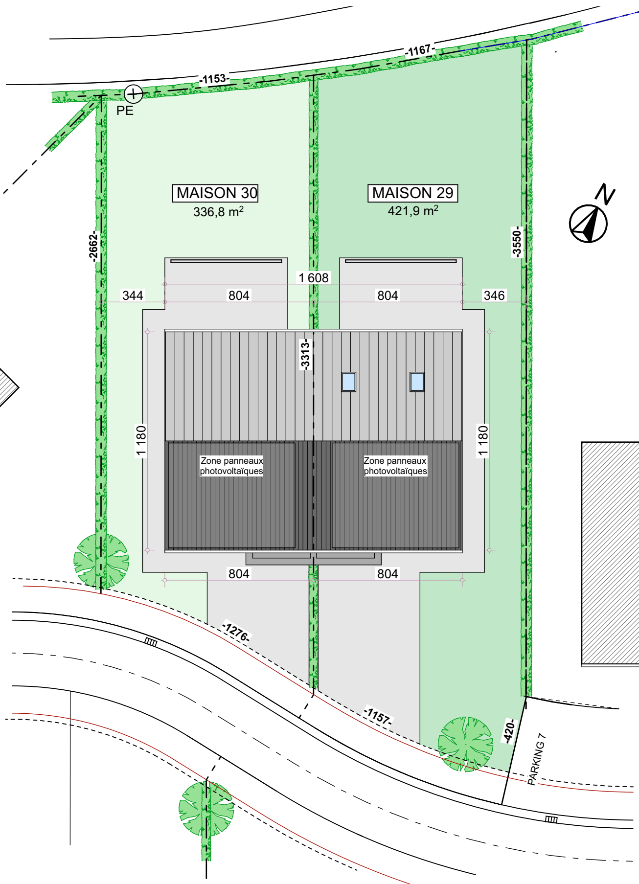
VERVIERS - STEMBERT - RUE HEPPINCHAMPS MAISONS 29 - 30 IMPLANTATION
