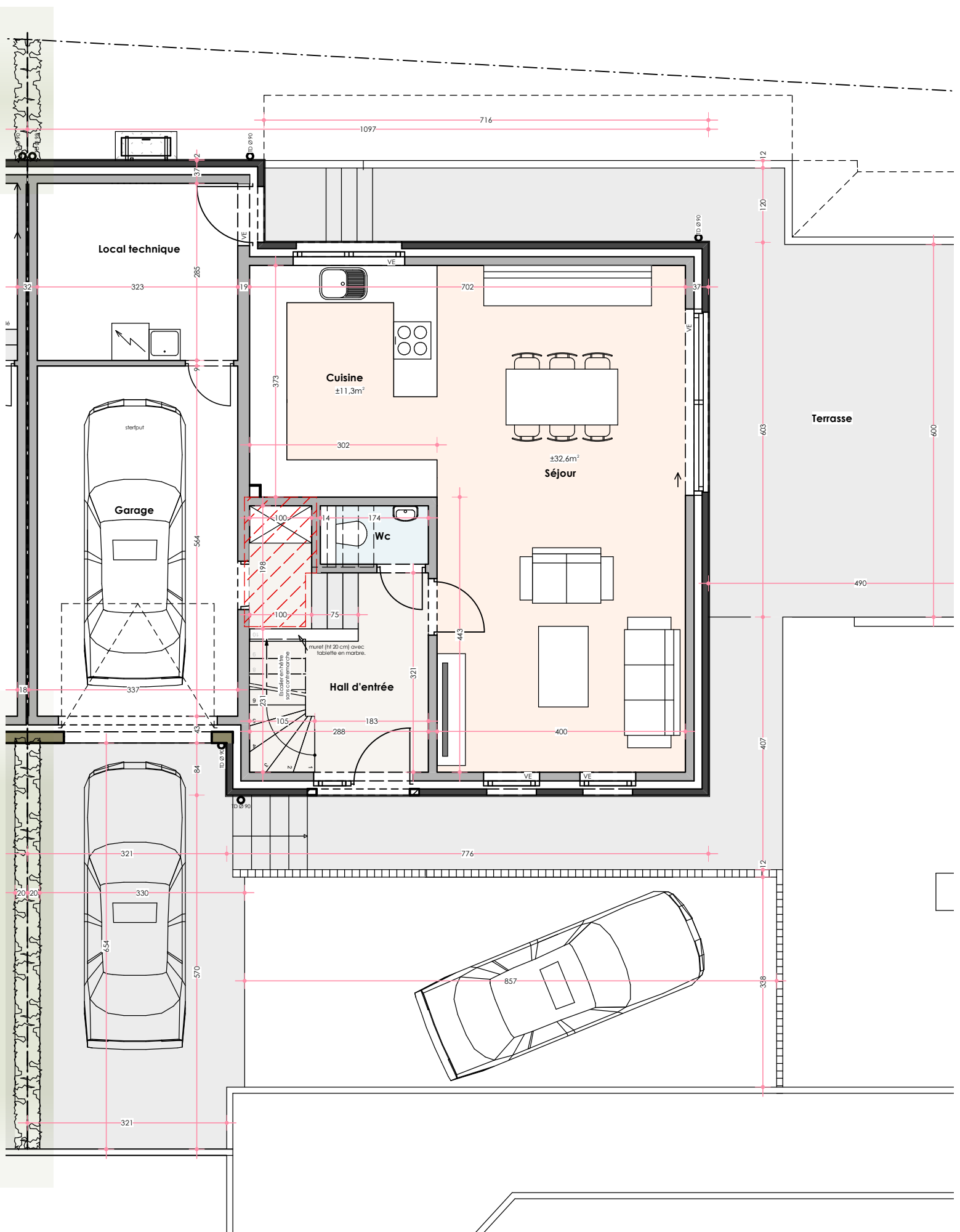
Maison 2 : Plan rez-de-chaussée
