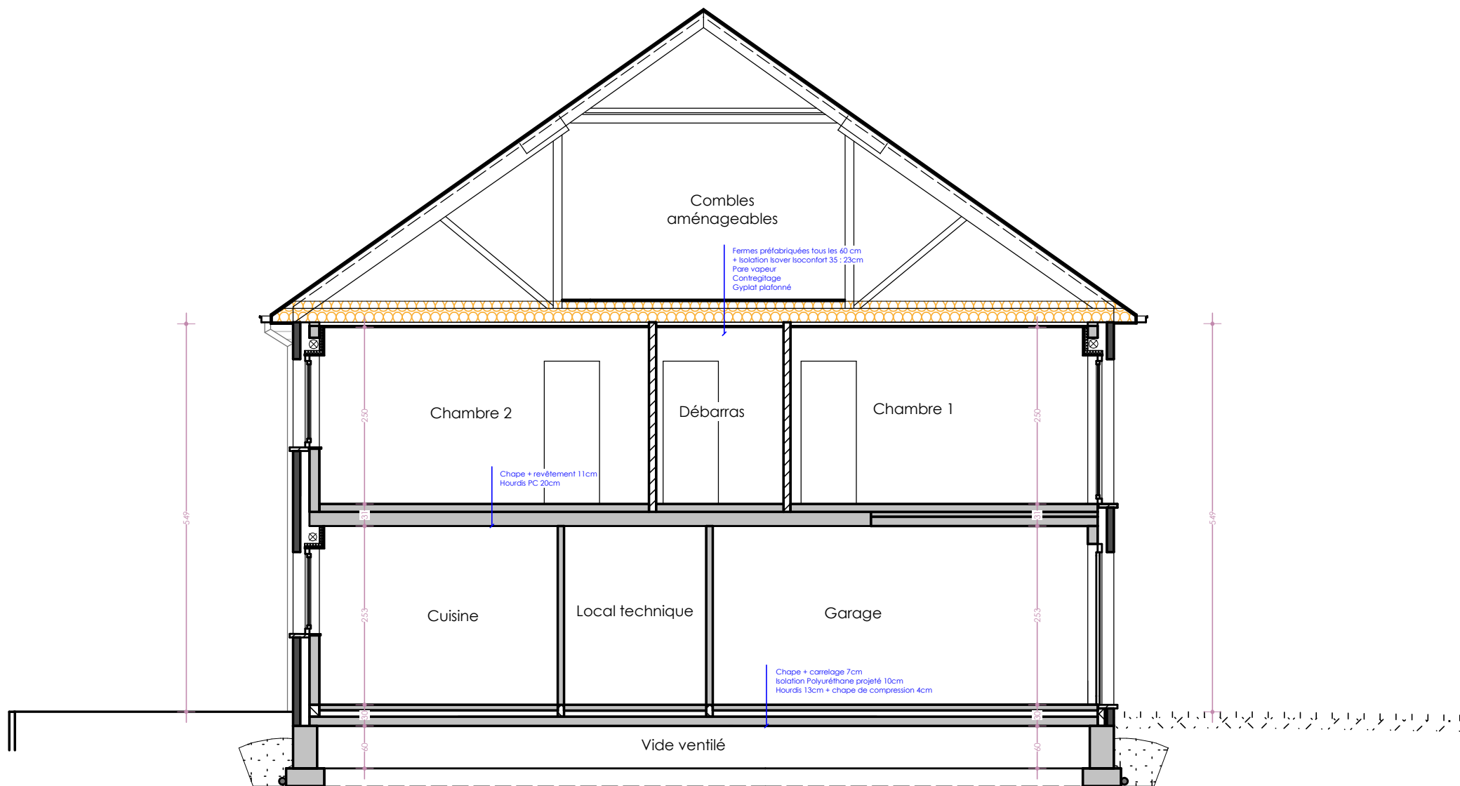
Coupe BB : Maison 36
